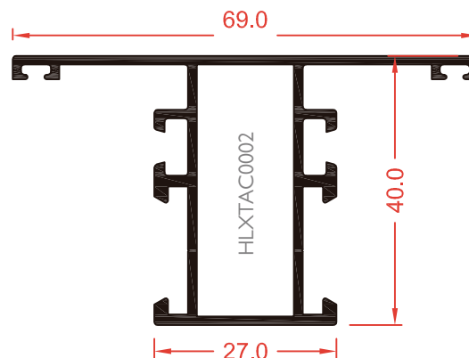
LEX5203 TRAVESAÑO 69 MM
