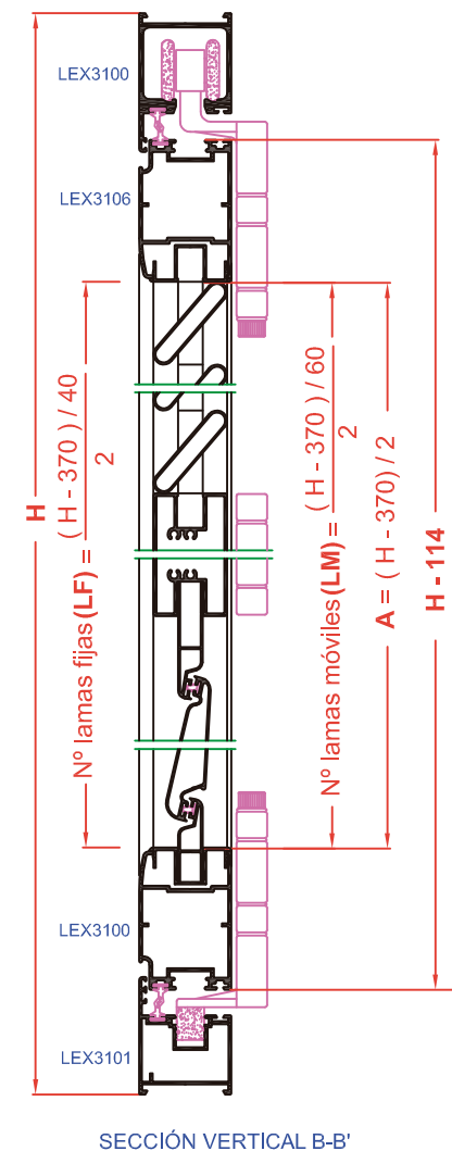
SECCIÓN VERTICAL B-B'
