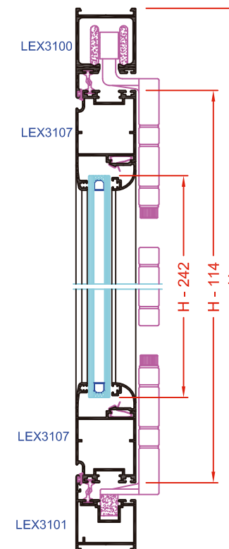
SECCIÓN VERTICAL B
