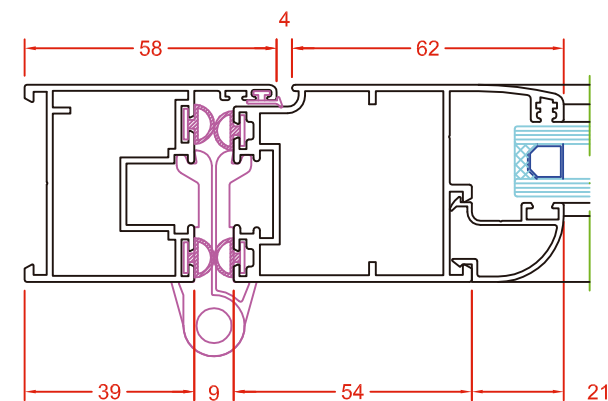
NUDO CENTRAL MARCO ACRISTALADA
