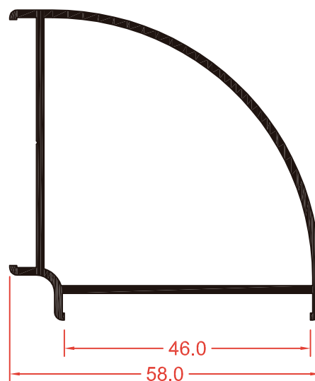
LEX9060 ESQUINERO 90 GRADOS
