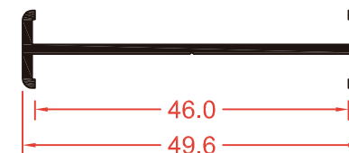
LEX9061 UNIÓN DE MARCOS
