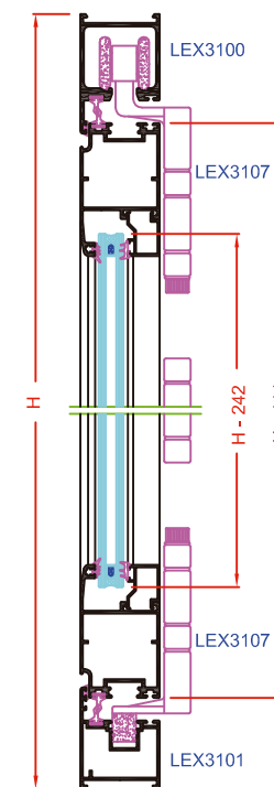
SECCIÓN VERTICAL B
