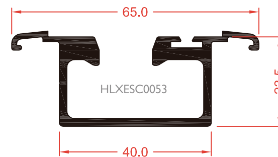
LEX3104 MARCO INFERIOR DE EMPOTRAR
