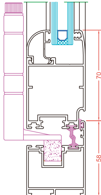
NUDO INFERIOR ACRISTALADA
