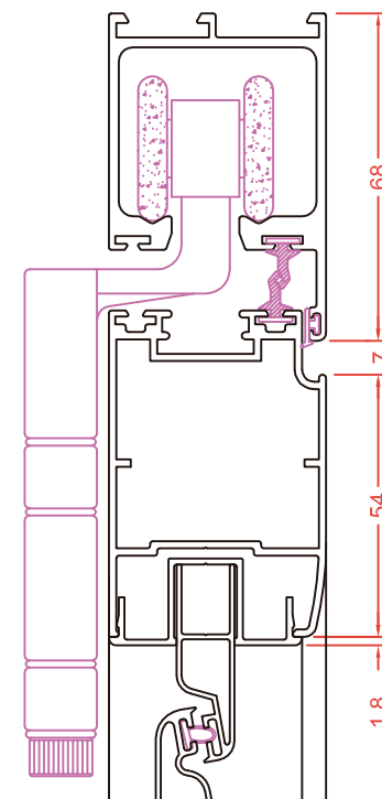
NUDO SUPERIOR MALLORQUINA
