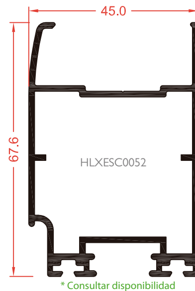
LEX3106 HOJA CURVA MALLORQUINA
