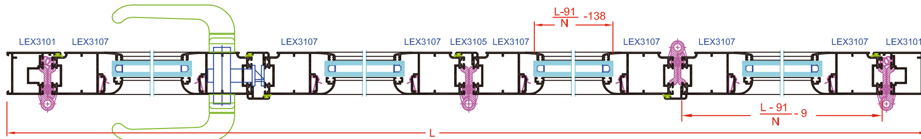
SECCIÓN HORIZONTAL A
