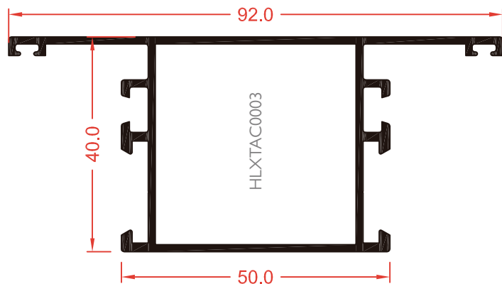
LEX5204 TRAVESAÑO 92 MM
