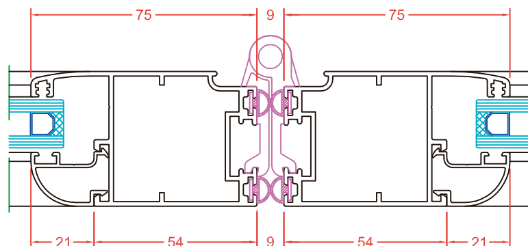
NUDO CENTRAL-BISAGRA EXTERIOR ACRISTALADA-OPCIÓN JUNTA Ó BATIENTE
