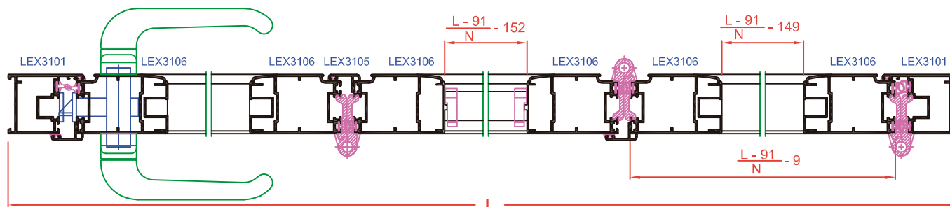
SECCIÓN HORIZONTAL A
