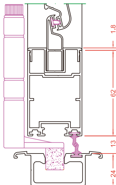
NUDO INFERIOR MALLORQUINA GUÍA EMPOTRADA
