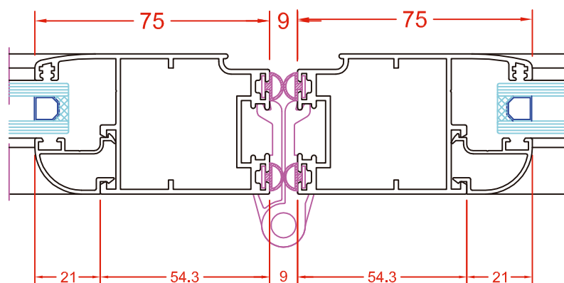
NUDO CENTRAL - BISAGRA INTERIOR ACRISTALADA-OPCIÓN JUNTA Ó BATIENTE
