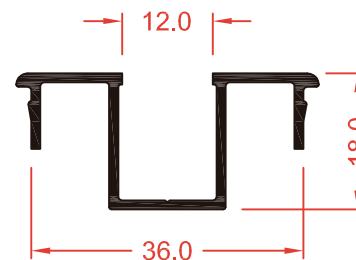
LEX10927 PERFIL BASE
