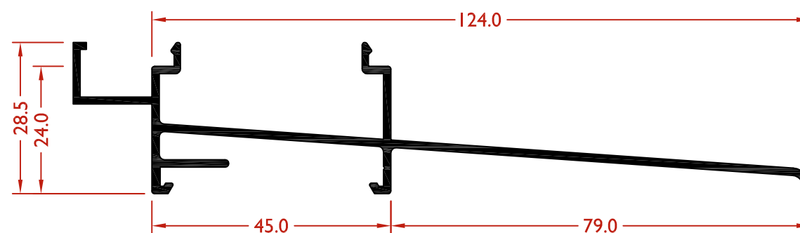
LEX9075 PERFIL DE CONDENSACIÓN CON VIERTEAGUAS
