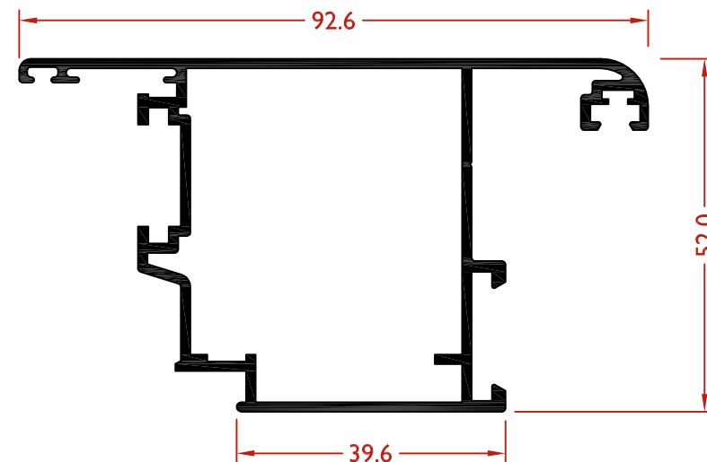
LEX9067 HOJA APERTURA EXTERIOR PUERTA
