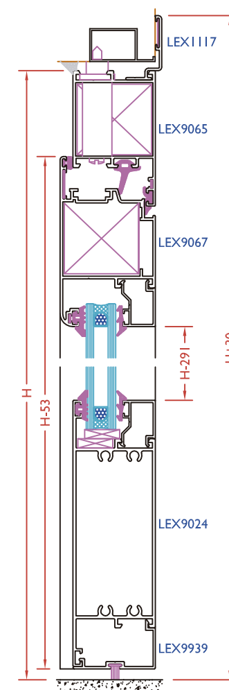
SECCIÓN B
