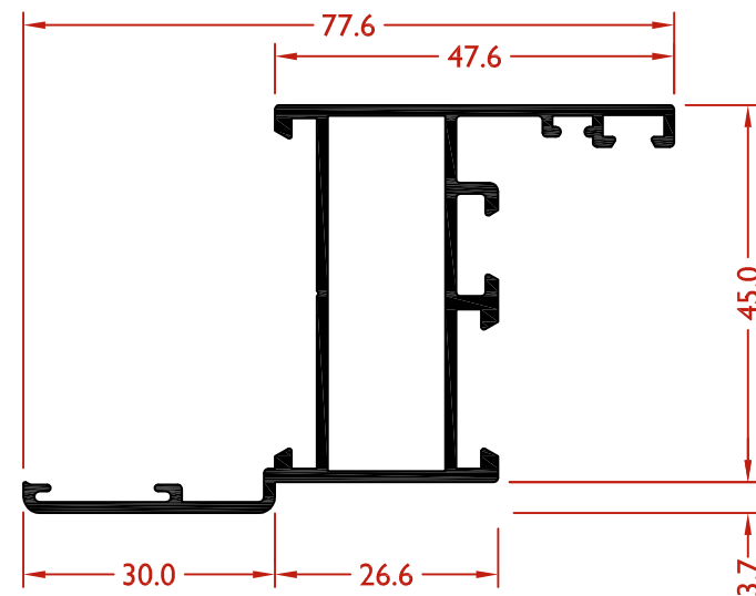
LEX9072 MARCO CON SOLAPE
