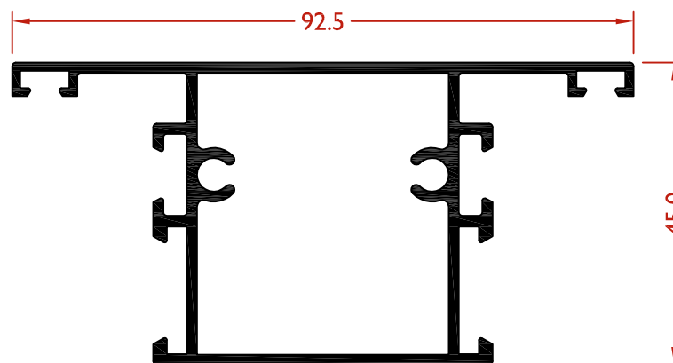
LEX9006 TRAVESAÑO 92,5 mm
