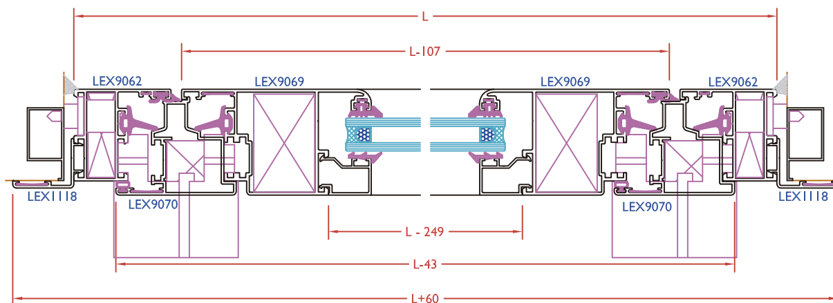
SECCIÓN A
