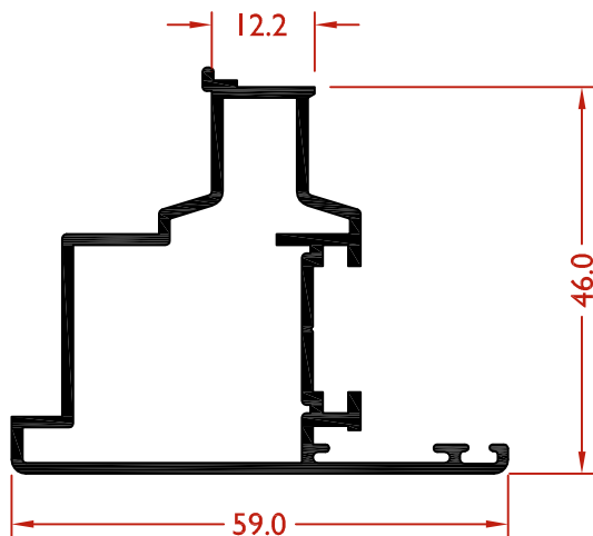
LEX9070 INVERSOR PIVOTANTE
