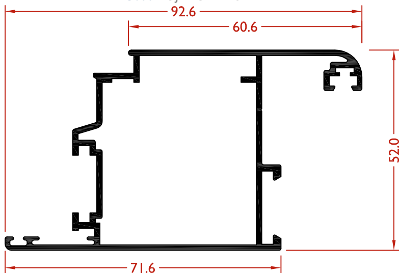
LEX9066 HOJA PUERTA 52 mm
