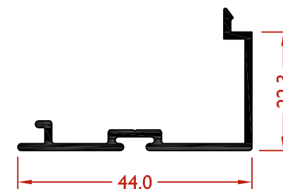
LEX9939 CIERRE INFERIOR ZÓCALO
