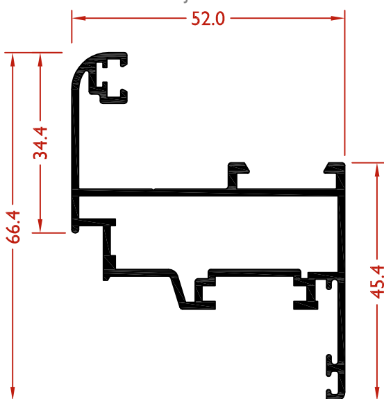
LEX9063 HOJA VENTANA 52 mm
