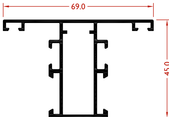
LEX9004 TRAVESAÑO 69 mm
