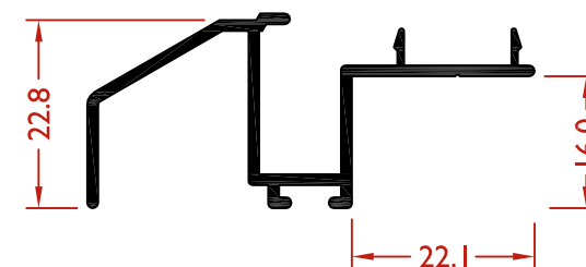
LEX9076 CIERRE INFERIOR HOJA
