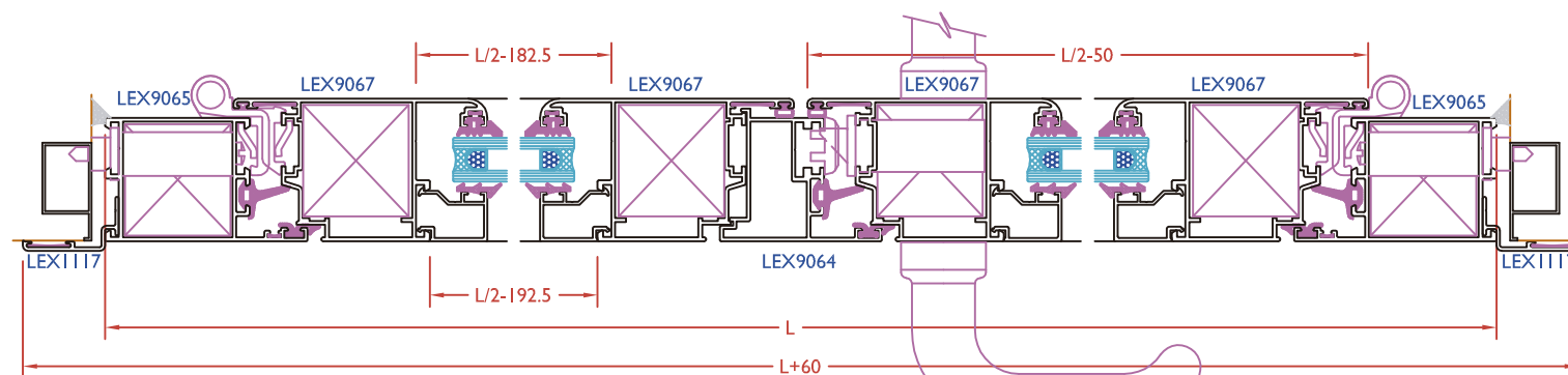
SECCIÓN A
