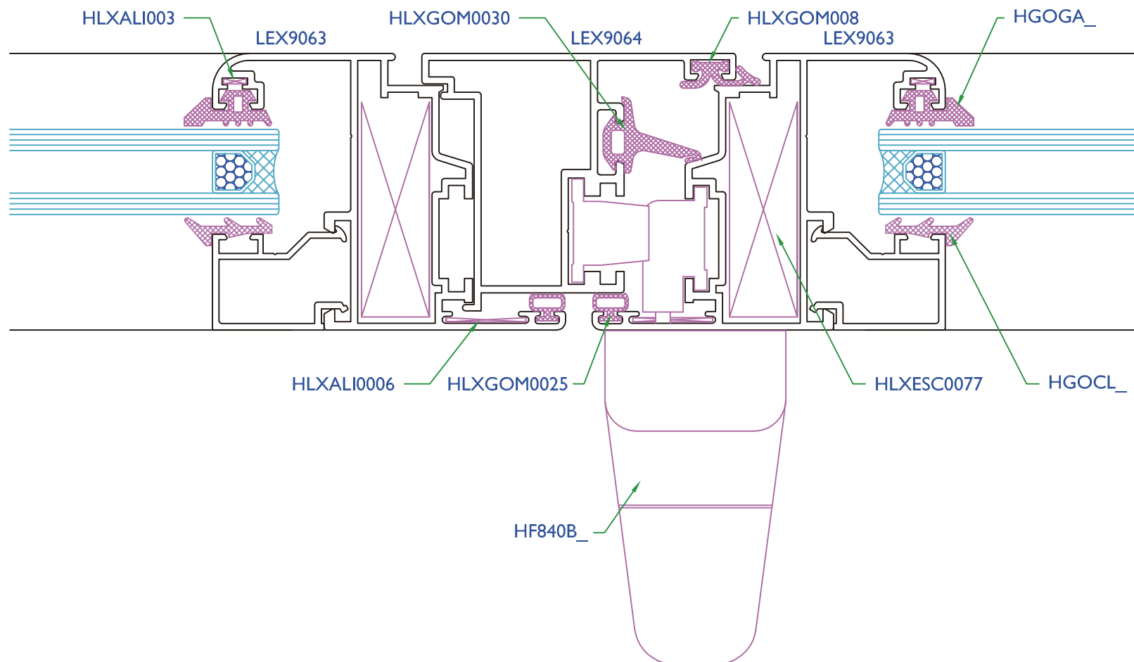
NUDO CENTRAL OSCIOBATIENTE
