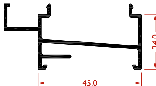
LEX9061 UNIÓN MARCOS
