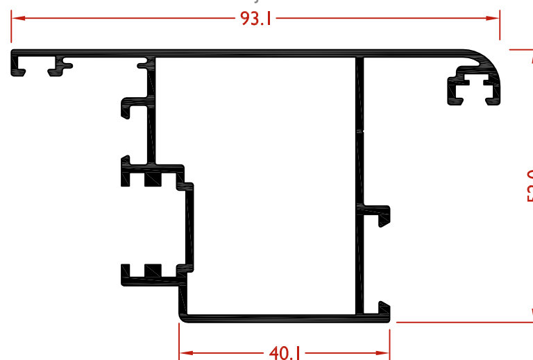
LEX9069 HOJA PIVOTANTE
