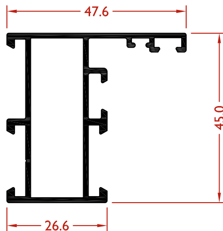
LEX9062 MARCO VENTANA 45 mm
