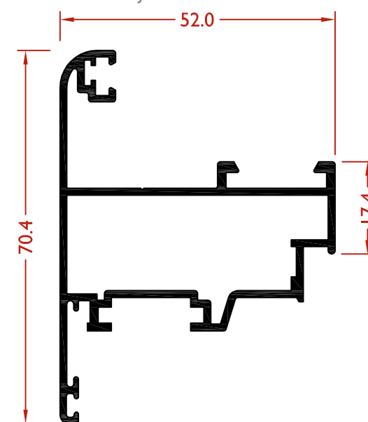
LEX9073 HOJA APERTURA EXT. VENTANA
